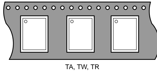
Figure 43. WLCSP 3-, 4-, 6-, 8-, 10-, & 12-Bump
